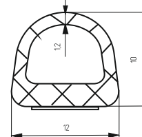
УПЛОТНИТЕЛЬ РГ-141 LT с клеевым слоем
