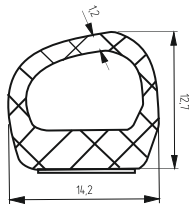
УПЛОТНИТЕЛЬ РГ-127-01 LT с клеевым слоем
