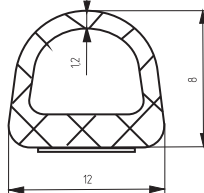
УПЛОТНИТЕЛЬ РГ-167В с усиленным клеевым слоем
