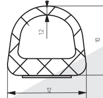
УПЛОТНИТЕЛЬ РГ-141В с усиленным клеевым слоем
