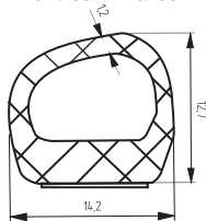
УПЛОТНИТЕЛЬ РГ-127-01 LT с клеевым слоем
