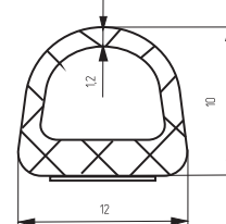
УПЛОТНИТЕЛЬ РГ-141 LT с клеевым слоем
